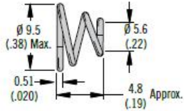
Ejector Spring
